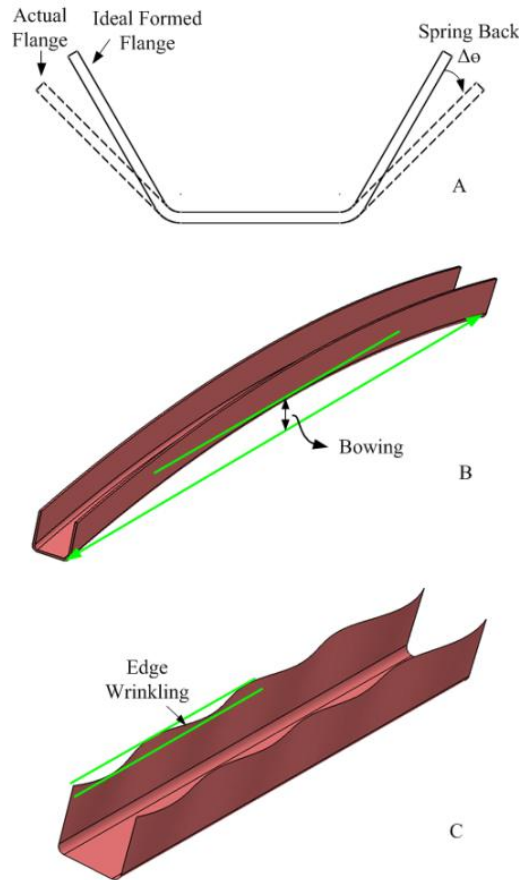
Fig. 4 Common defects in roll forming process of channel sections, A) Spring back, B) Bowing and C) edge wrinkling شکل 4 عیوب هندسی متداول در شکل‌دهی غلتکی، A) عیب برگشت فنی، B) عیب کمائی شده و C) عیب موج لبه
