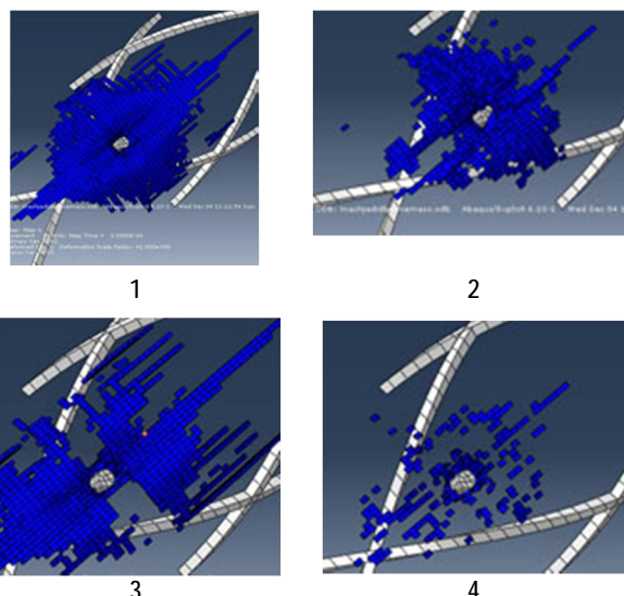
شکل 16 گستردگی سطح آسیب‌دیدگی
