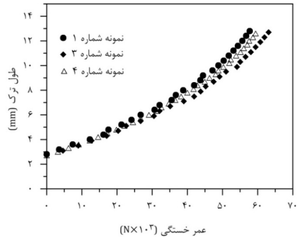
شکل 9 نتایج تجربی آزمون رشد ترک نمونه استاندارد از فولاد AISI 4140
