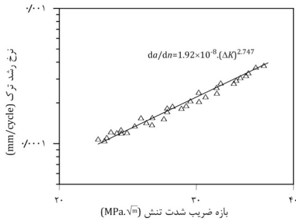
شکل 9 نتایج تجربی آزمون رشد ترک نمونه استاندارد از فولاد AISI 4140
