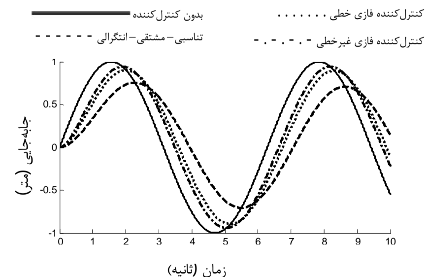
شکل 17 خروجی سیستم فازی خطی و غیرخطی به‌ازای ورودی سینوسی
