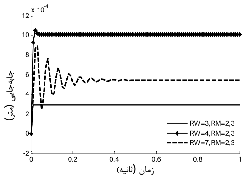
شکل 15 مقایسه دامنه ارتعاشات کنترل شده ورق مستطیلی چهارلایه مستقر بر بستر خطی تحت نیروی اجباری در موقعیت‌های متفاوت
