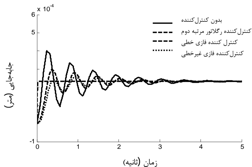
شکل 16 مقایسه پاسخ زمانی سه نوع کنترل کننده ارتعاشات ورق مستطیلی مستقر بر بستر خطی تحت نیروی اجباری پله
