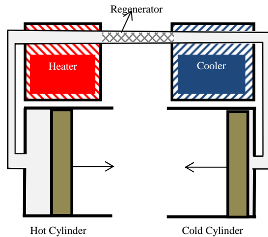
Fig. 2 The schematic of Alpha type of Stirling configurations [19] شکل 2 طرحواره موتور استرلینگ نوع آلفا [19]
