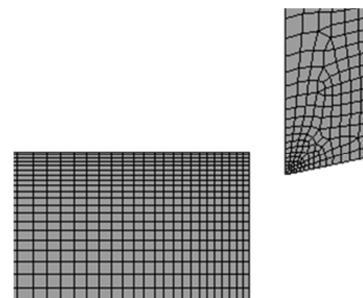
شکل ۴ مدل ایجاد شده برای ابزار کاربیدی و قطعه کار در شبیه‌سازی اجزاء محدود
