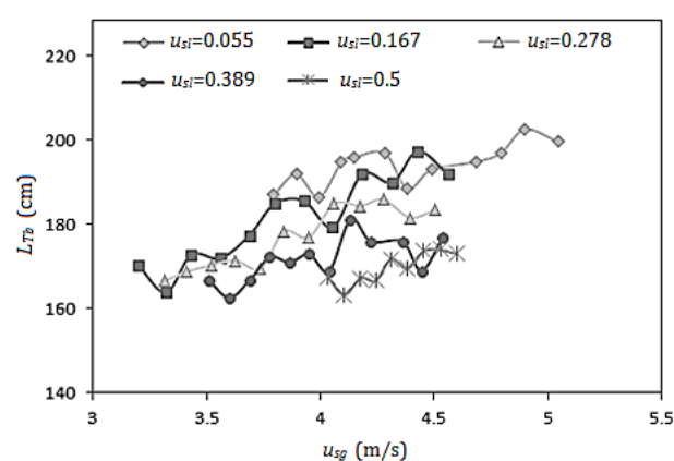
شکل 14 تغییرات طول متوسط حباب‌ها در شیب سوم
