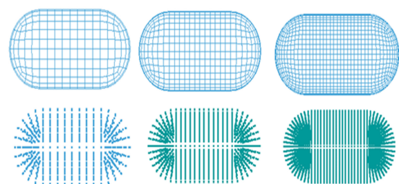
شکل ۷ شبکه‌بندی لاگرانژ و SPH مدل پرنده با سه اندازه شبکه
