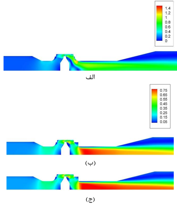
شکل ۱۰) تغییرات عدد ماخ برای شرایط الف) بدون ساینسر، ب) با ساینسر ۲۰ ppi، ج) با ساینسر ۱۰ ppi
