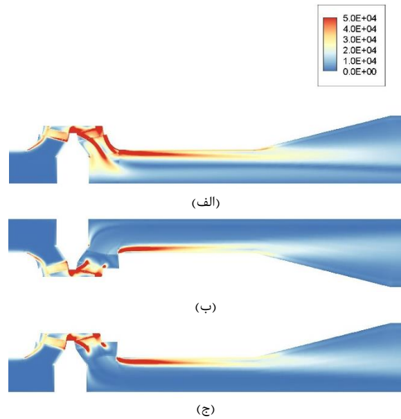
شکل ۱۳ تغییرات ورتیسیت (1/sec) برای شرایط الف) بدون ساینسر، ب) با ساینسر ۱۰ ppi، ج) با ساینسر ۲۰ ppi
