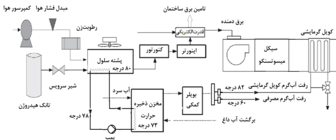
شکل ۱ پکیج تولید چندگانه بر اساس پیل سوختی پلیمری
