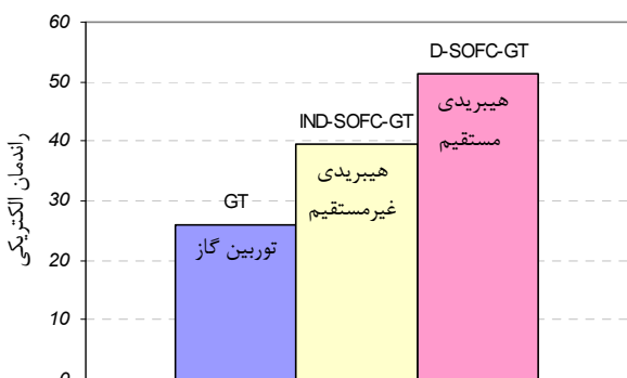
شکل ۲۲ مقایسه راندمان الکتریکی سیستم‌های هیبریدی
