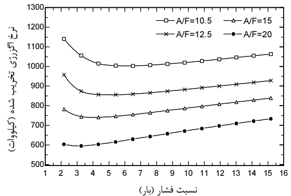
شکل ۱۱ تأثیر نسبت فشار دمپرسور بر روی نرخ انرژی تخریب شده در سیستم هیبریدی
