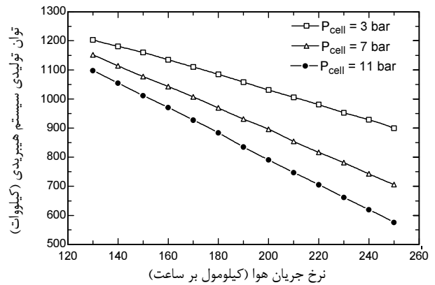
شکل ۱۵ تأثیر نرخ جریان هوای ورودی به سیستم بر روی نرخ انرژی تخریب شده (کیلووات)
