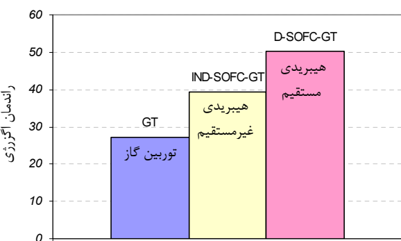
شکل ۲۳ مقایسه راندمان آگرژی سیستم‌های هیبریدی
