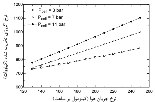
شکل ۱۶ تأثیر نرخ جریان هوای ورودی به سیستم بر روی نرخ انرژی تخریب شده (کیلووات)
