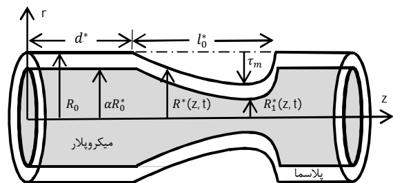
شکل 1 هندسه جریان خون دوبعدی در سرخرگ گرفته شده
