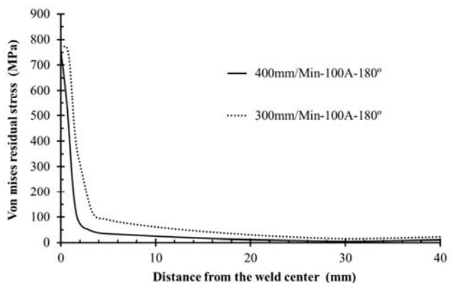
Fig. 20 Von Mises residual stress in the 100A current شکل 20 تنش پسماند فون میسز در شدت جریان 100 آمپر
