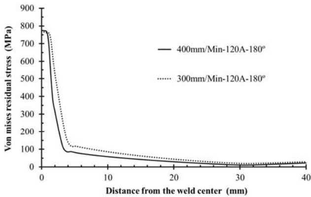
Fig. 21 Von Mises residual stress in the 120A current شکل 21 تنش پسماند فون میسز در شدت جریان 120 آمپر
