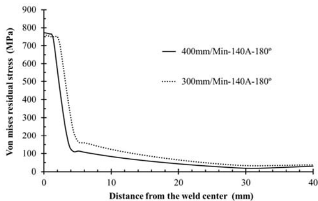
Fig. 22 Von Mises residual stress in the 140A current شکل 22 تنش پسماند فون میسز در شدت جریان 140 آمپر
