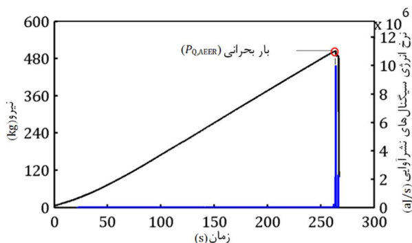
شکل 15 تعیین بار بحرانی به روش نرخ انرژی سیگنال‌های نشر آوابی در نمونه C
