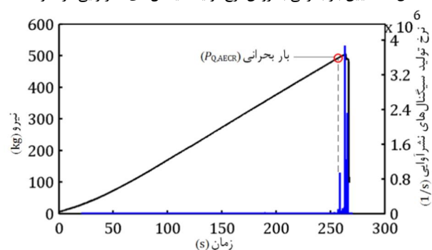
شکل 12 تعیین بار بحرانی به روش نرخ تولید سیگنال‌های نشر آوابی در
