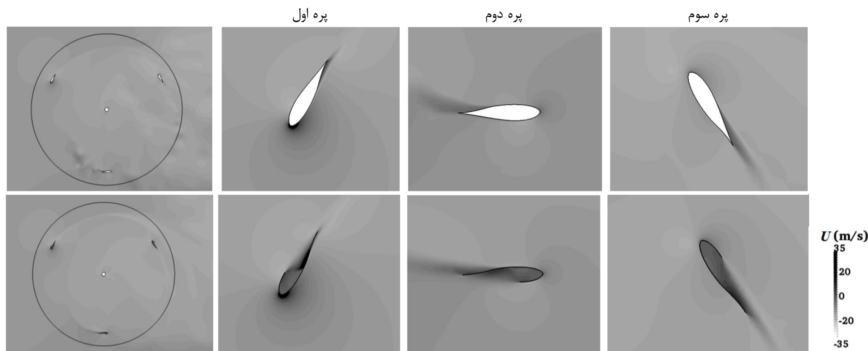
شکل 21 میدان سرعت حول روتور و پره‌ها پس از رسیدن به حالت پایا در یک دوران کامل برای پره با ایرفویل Du 06-W-200 و J-33 Du در سرعت نوک بهینه
