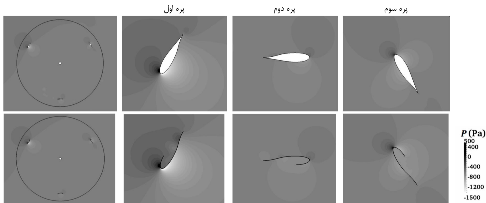
شکل 22 میدان فشار حول روتور و پره‌ها پس از رسیدن به حالت پایا در یک دوران کامل برای پره با ایرفویل Du 06-W-200 و J-33 Du در سرعت نوک بهینه
