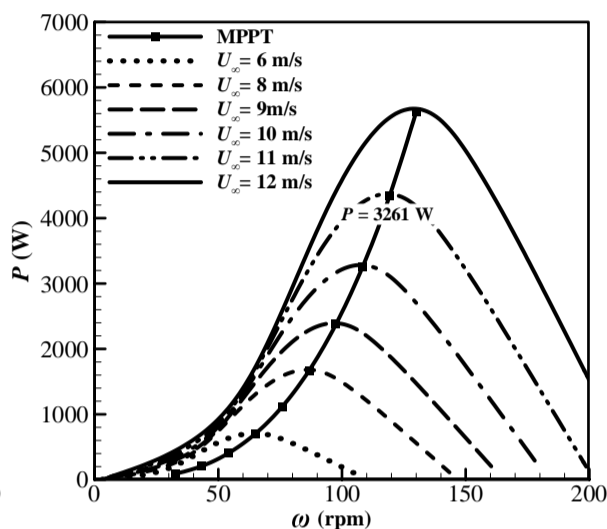
شکل 16 منحنی توان و MPPT برای پره با مقطع Du 13- شکل 17 منحنی توان و MPPT برای پره با مقطع Du 23- شکل 18 منحنی توان و MPPT برای پره با مقطع Du 33- شکل 19 منحنی توان و MPPT برای پره با مقطع Du 43- شکل 20 منحنی توان و MPPT برای پره با مقطع Du 53-
