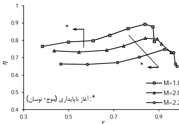
شکل 5 نمودار عملکردی ورودی در اعداد ماخ 1/8، 2/0 و 2/2
