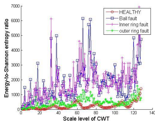
Fig. 4 Optimum Scales
