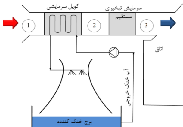
شکل ۱ شماتیک سیستم سرمایش ترکیبی برج خنک کننده و سرمایش تبخیری مستقیم
