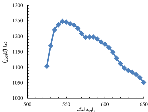
شکل 8 دمای نقطه‌ای گازهای عبوری از درگاه خروجی (شبیه‌سازی)
