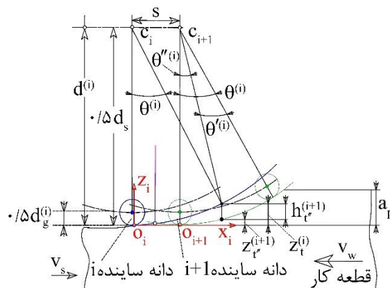
شکل ۴) آنالیز سینماتیکی مسیر حرکت چندین دانه ساینده
