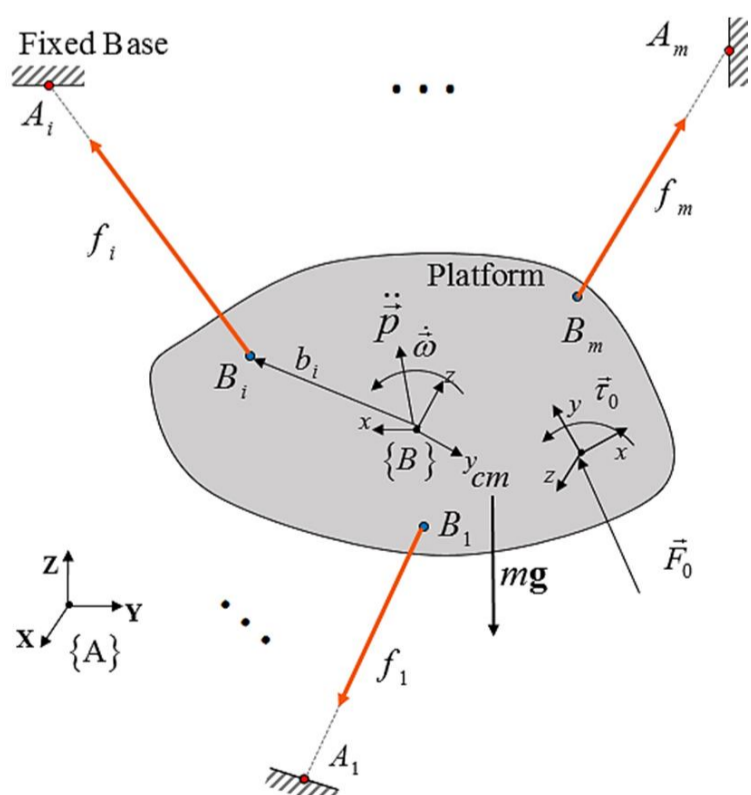
Fig. 3 Dynamics parameter of the hybrid robot
