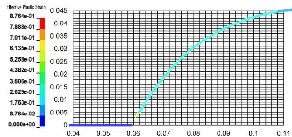
شکل ۱۵) آسیب ورق ۱ میلی‌متر تحت انفجار با فشار اولیه ۵ بار
