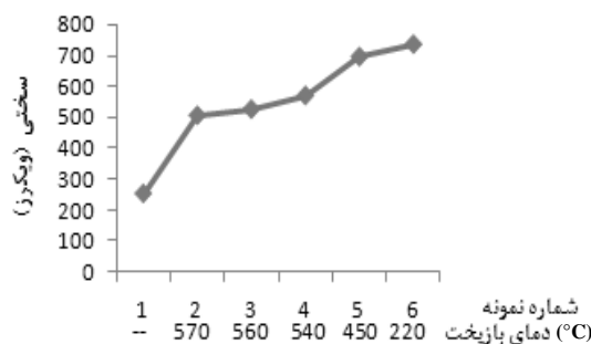
شکل ۵ تاثیر دمای بازیخت بر روی سختی نمونه‌ها
