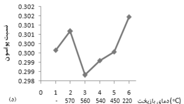
شکل ۷ تاثیر دمای بازپخت بر روی خواص مکانیکی نمونه‌های فولاد AISI D6: (الف) مدول برشی (ب) مدول یانگ (ج) مدول حجمی (د) نسبت پواسون
