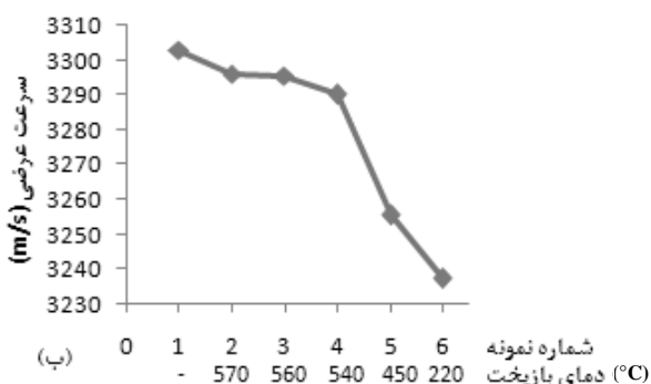
شکل ۶ خواص فراصوتی نمونه‌های فولاد AISI D6، (الف) سرعت طولی (ب) سرعت عرضی
