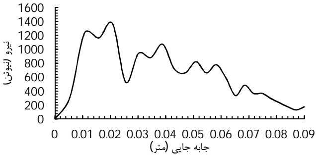
شکل 20 نمودار نیرو - جابه‌جایی نمونه مشبک 1-1
