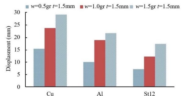
Fig. 19 Maximum experimental deflection of circular plate's with 1.5mm thickness by different explosive charges in different materials شکل 19 حداکثر تغییر شکل تجربی مرکز ورق دایروی با ضخامت 1.5 میلی‌متر برای خرج‌های انفجاری مختلف در جنس‌های متفاوت
