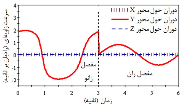
شکل 10 نمودار سرعت زاویه‌ای
