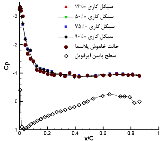
شکل ۸ توزیع فشار حول ایرفویل در زاویه حمله ۲۰ درجه در حالت‌های عملگر روشن با فرکانس 100\text{ Hz} (سیکل‌های کاری متفاوت) و عملگر خاموش
