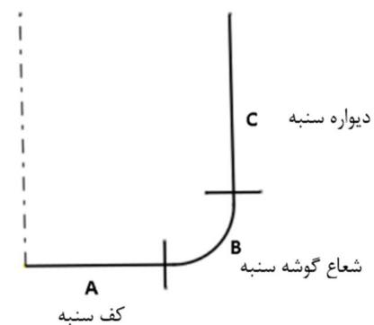
شکل 10 ناحیه بندی قطعه کار برای بررسی توزیع ضخامت
