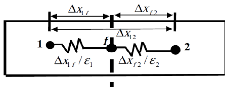
شکل ۲ ناحیه محاسباتی و شرایط مرزی برای معادله (۸)
