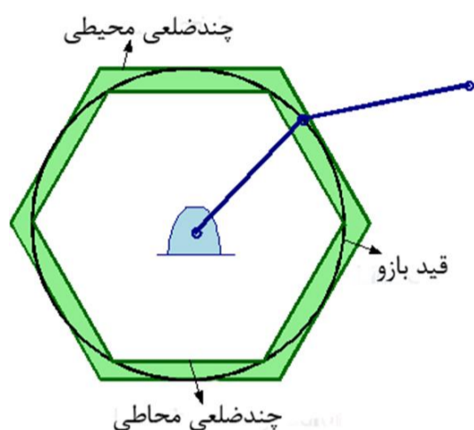
شکل 6 نمایش چند ضلعی‌های محیطی و محاطی تقریب زده شده برای قیدهای سینماتیکی [13]
