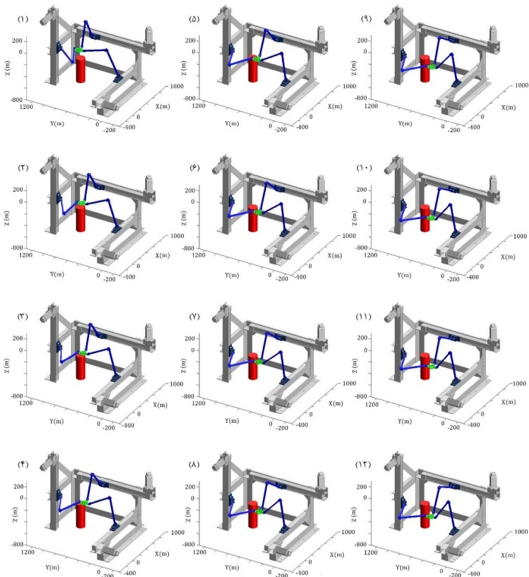
شکل 10 فریم‌هایی از فیلم شبیه‌سازی الگوریتم مسیریابی بر روی مدل واقعی ربات موازی تریپترون با شرایط جدول 3 و با تابع هزینه کوتاه‌ترین مسیر در حضور مانع ثابت
