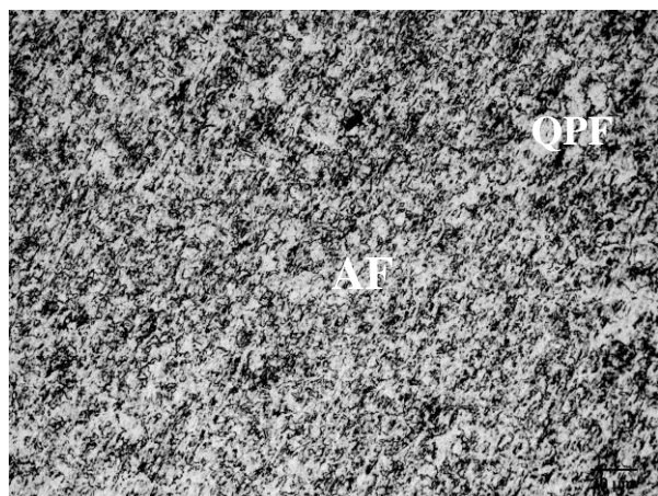
شکل ۶ ریزساختار فولاد ایکس ۶۵ در سرعت سرد کردن 5^{\circ}\text{C/s} (شکل ۶) فریت شبه چند وجهی، AF فریت سوزنی).
