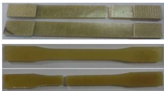
شکل 5 نمونه آزمایش کشش رزین و الیاف عرضی
