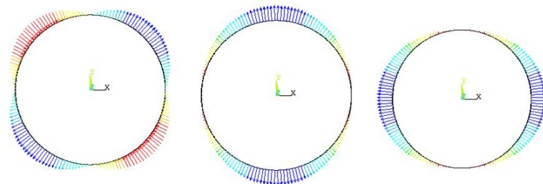
شکل 6 نحوه اعمال بارگذاری شعاعی الف) \sigma_x = 1 ب) \sigma_y = 1 ج) \sigma_{xy} = 1
