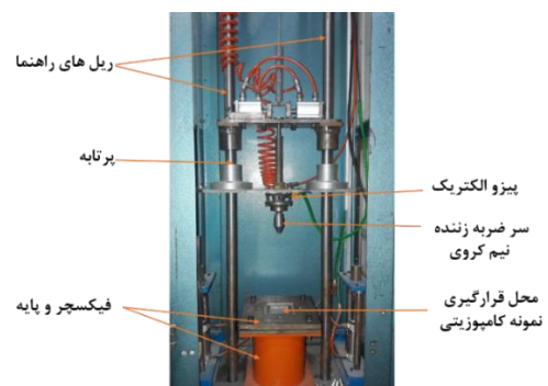
شکل ۲) نمایی از دستگاه آزمون ضربه کم سرعت
