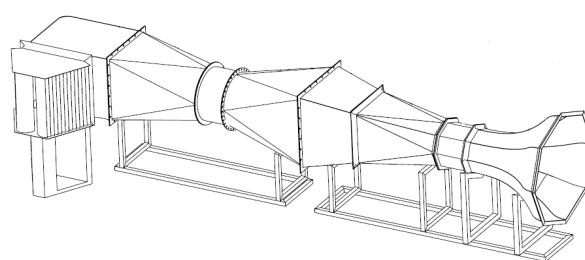
شکل ۳ تونل باد مدار باز مکنده
