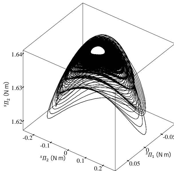
شکل 11 مسیر بردار مومنوم زاویه‌ای ماهواره بیان شده در دستگاه مختصات ماهواره پس از هم‌گرایی به منیفولد مرکزی (از 40 تا 1000 مدار)
