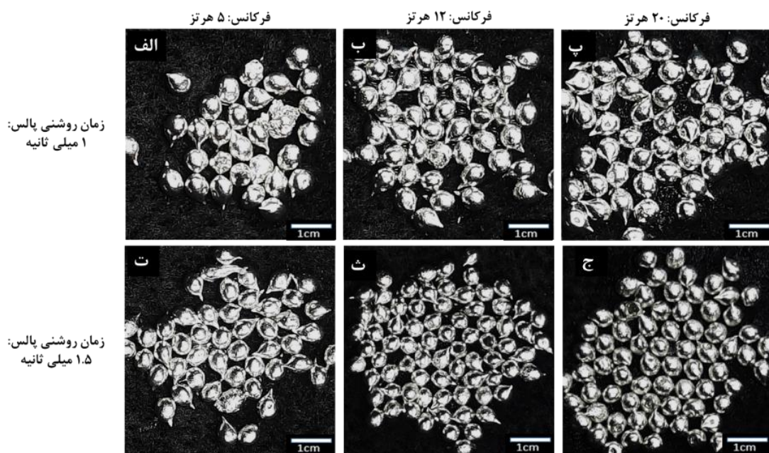
شکل ۴) نتایج حاصل از تغییر بسامد و زمان روشنی پالس قلع خالص در ولتاژ ۲۸۰ ولت و در دمای ۳۲۰ درجه سانتی‌گراد
