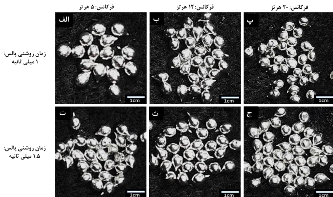
شکل ۳) نتایج حاصل از تغییر بسامد و زمان روشنی پالس قلع خالص در ولتاژ ۲۰۰ ولت و در دمای ۳۲۰ درجه سانتی‌گراد
