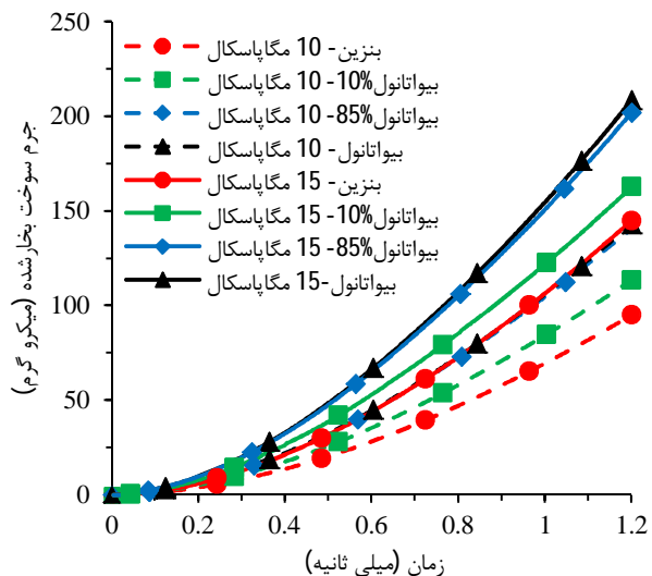
شکل 11 مقایسه‌ی جرم سوخت بخار شده در حین تزریق با افزایش فشار تزریق از 10 مگاپاسکال به 15 مگاپاسکال
