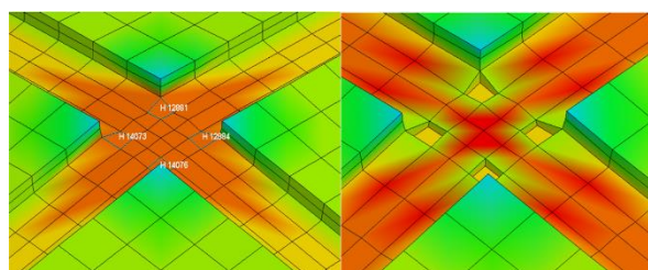
شکل ۷) محدوده شروع پارگی دیسک فداشونده با عمق شیار ۰/۵ میلی‌متر
