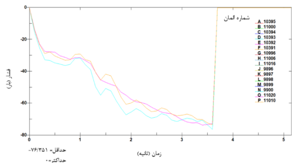
شکل ۸) نمودار فشار-زمان برای شروع پارگی دیسک فداشونده در عمق شیار ۰/۴ میلی‌متر
