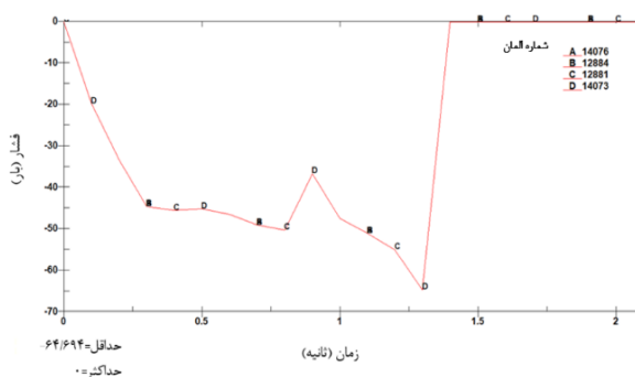
شکل ۹) نمودار فشار-زمان برای شروع پارگی دیسک فداشونده در عمق شیار ۰/۵ میلی‌متر
