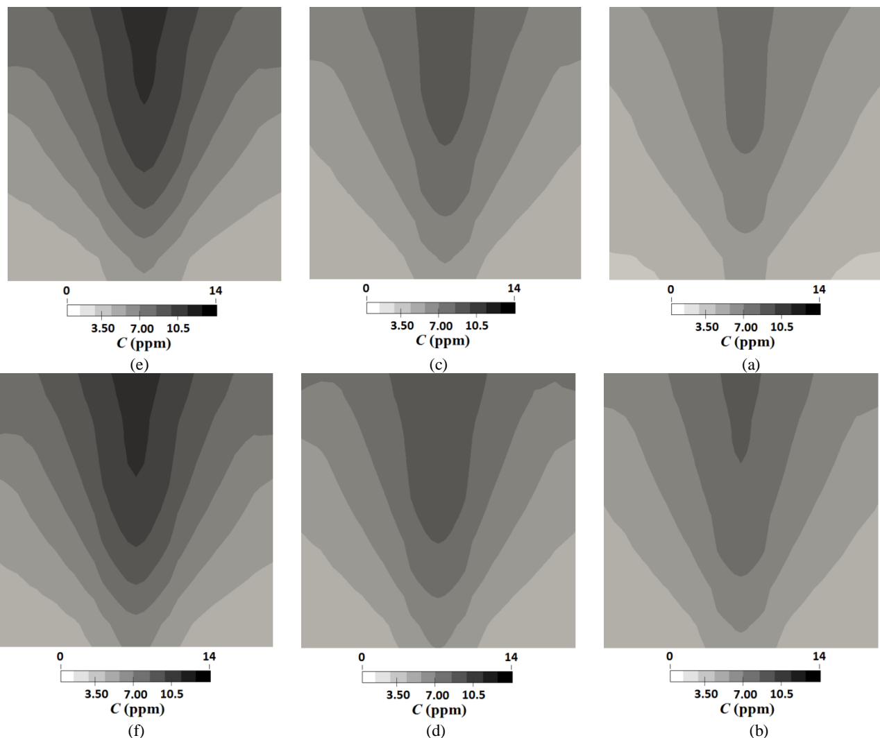
Fig. 5 Counter of pollutant concentration of back wall of building for reference velocity of 4.7 m/s for case No. (a) 4, (b) 1, (c) 5, (d) 2, (e) 6 and (f) 3 شکل 5 کانتور توزیع غلظت آلاینده بر روی دیوار پشتی ساختمان برای سرعت مرجع 4.7 متر بر ثانیه در شبیه‌سازی شماره: (a) 4، (b) 1، (c) 5، (d) 2، (e) 6 و (f) 3
