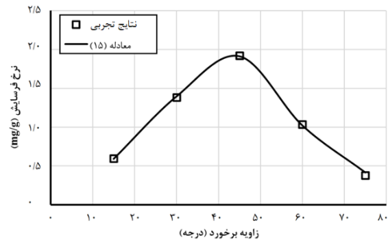
شکل ۹) مقایسه نتایج حاصل از نتایج تجربی و مدل پیش‌بینی از معادله (۹) در سرعت ۱۲۰ متر بر ثانیه
