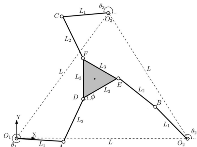
شکل 1 ربات موازی صفحه‌ای 3-RRR و نام گذاری اجزا آن
