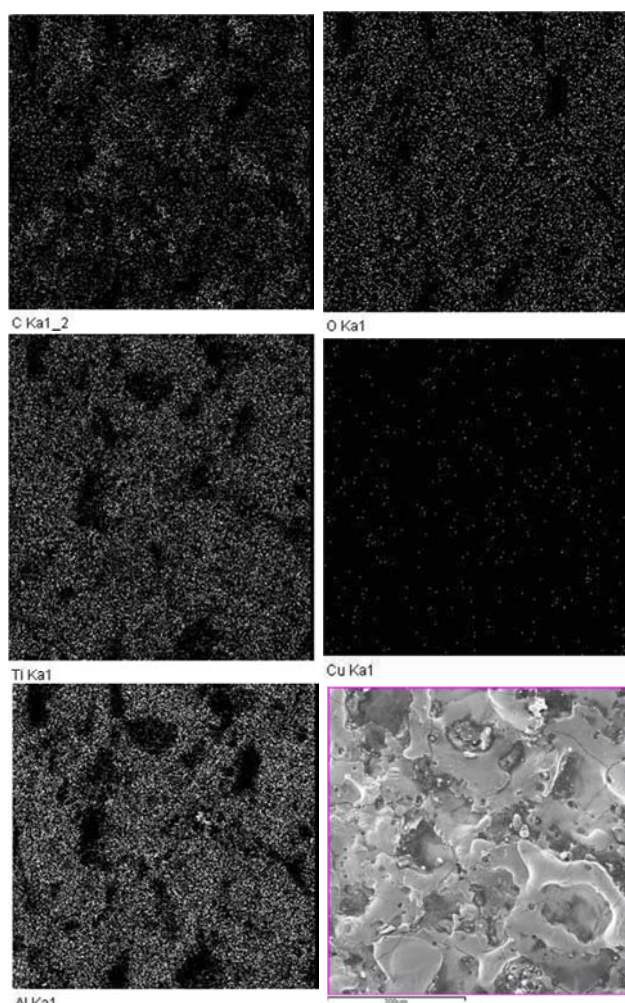
شکل ۷ آنالیز EDS-Map بر روی سطح ماشینکاری شده با استفاده از الکتروُد مس
