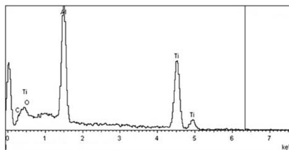
شکل ۱۱ آنالیز EDS موضعی مربوط به قسمت روشن تر در نمونه ماشینکاری شده با الکتروود مس
