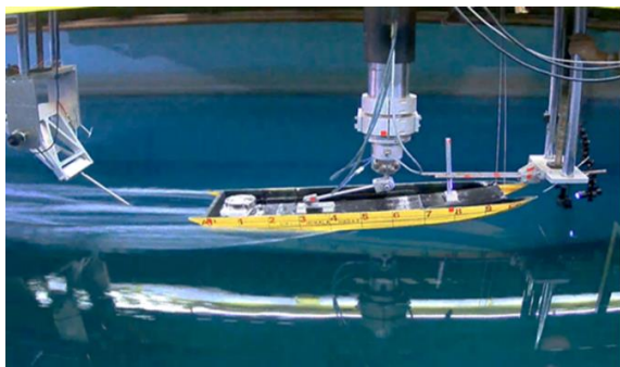
شکل (۲) آزمایش شناور در حوضچه کشتی آزمایشگاه دریایی خلیج فارس در عدد فرود طولی ۱/۵۵
