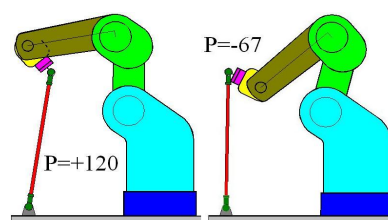
شکل ۷ وضعیت حدی مفصل P
