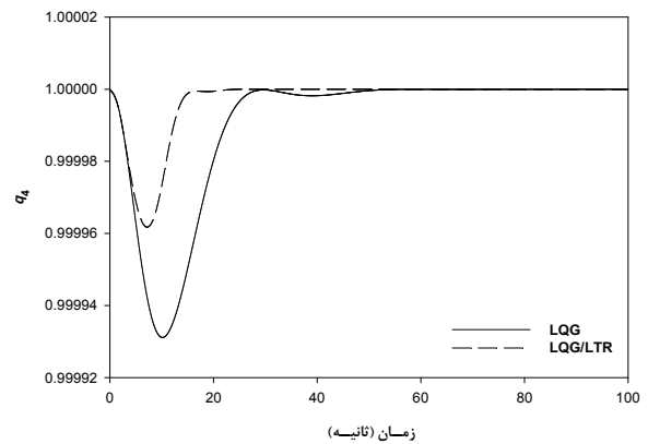
شکل ۹ مولفه q_4 کوآرنیون های وضعیت LQG و LQG/LTR
