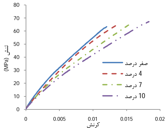
شکل 7 نمودار تنش-کرنش در کشش الیاف عرضی
