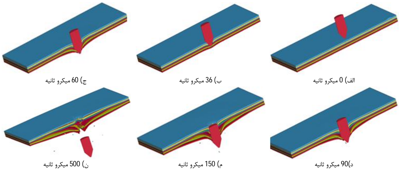
شکل 11 نتیجه شبیه‌سازی پرتابه در زمان نفوذ
