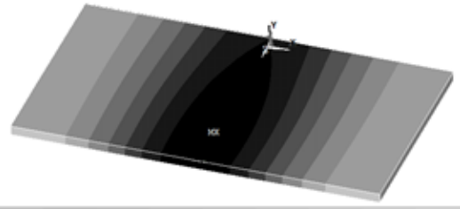
شکل ۴ توزیع حرارتی نمونه بعد از خنک شدن (اعداد بر حسب درجه سانتی گراد)
