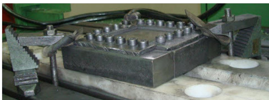
شکل 5 فیکسچر ساخته شده برای شکل‌دهی ورق Ti-6Al-4V
