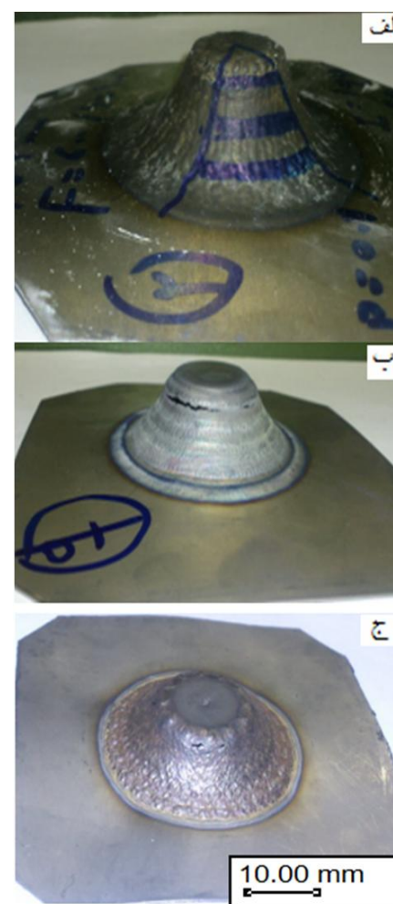
شکل 19 قطعات تولیدشده با حداکثر زاویه‌ی شکل‌دهی از ورق Ti-6Al-4V با
