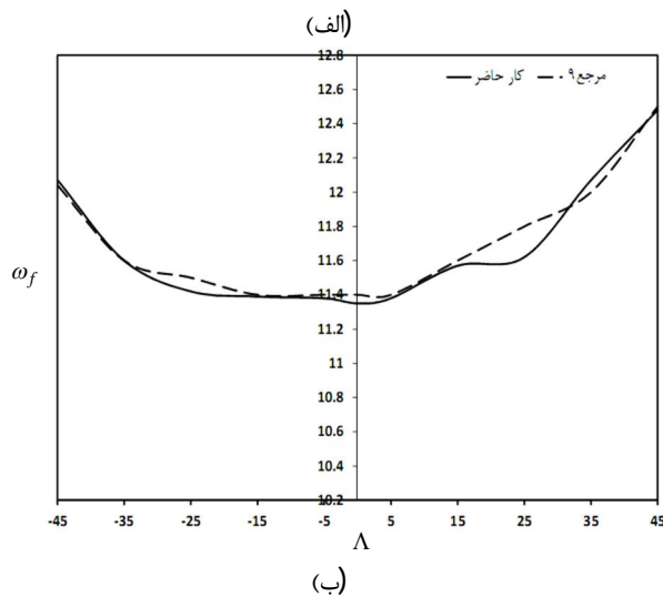
شکل 6 اثر تغییر زاویه عقبگرد بال تنها بر روی (الف) سرعت فلاتر و (ب) فرکانس فلاتر 2
